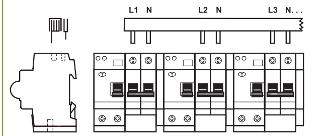
PS 4/40/16-DDA 204 T DS 204 (≤ 40 A) + DS 204 (≤ 40 A) + DDA 204 (≤ 40 A) + S 204 + DDA 204 (≤ 40 A) + S 204 ...
