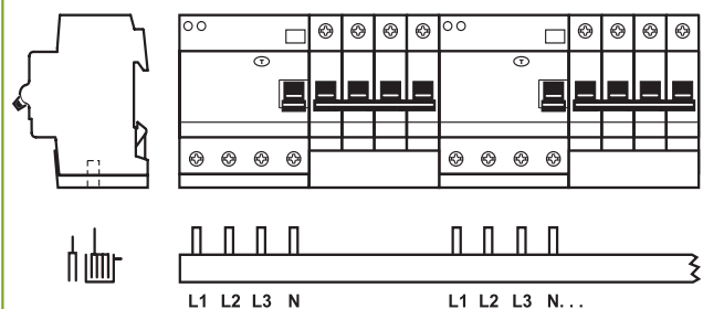
PS 3/30/16-DDA 202 T DS 202 + DS 202 + DA 202 + S 202 + DDA 202 + S 202 ...
