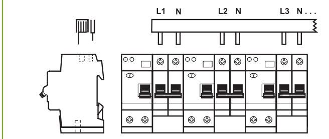
PS 4/30/16N-DDA 202 T DS 202 + DS 202 + (DDA 202 + S 202) ...
